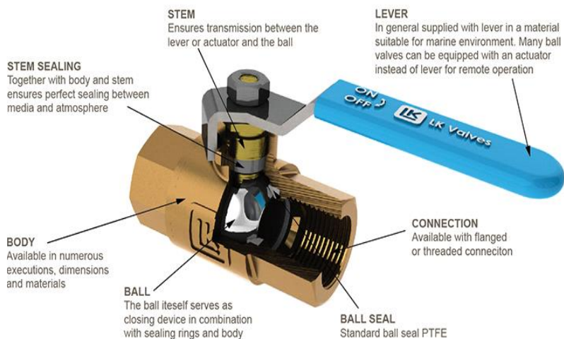
Figura 44. Esempio di valvola a sfera
