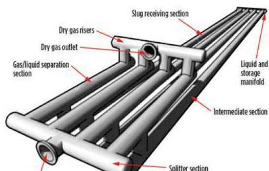
Figura 15. Separatore di tipo Slog catcher
