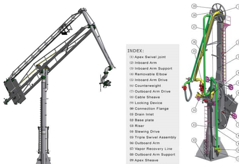
Figura 39. Bracci di carico marini per il rifornimento di GNL: layout e componenti
