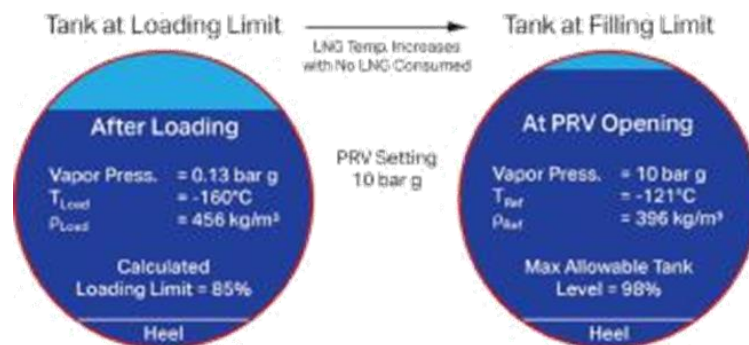
Figura 54. Limite di caricamento per un tipico serbatoio pressurizzato
