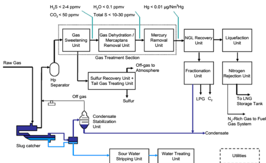
Figura 2 Schema di un impianto per la produzione di GNL
