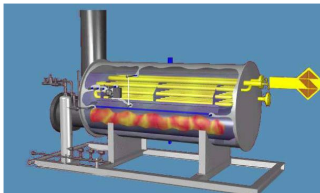
Figura 17. Forno a fiamma indiretta
