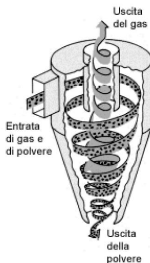
Figura 16. Separatore ciclonico
