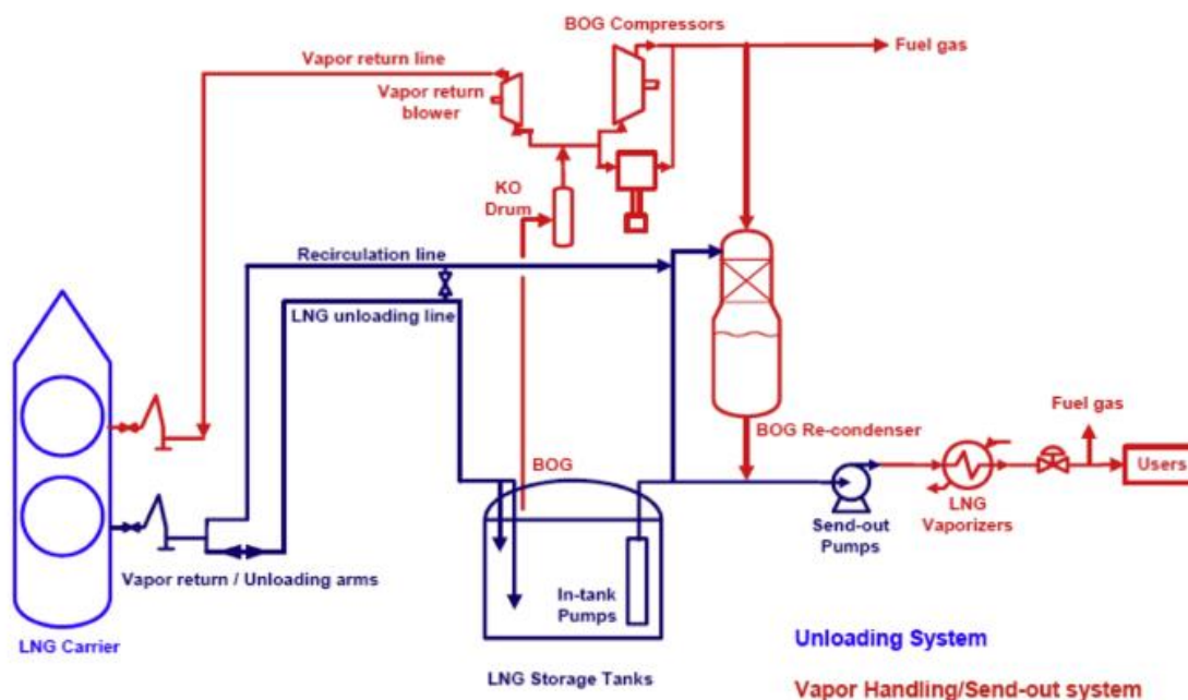
Figura 4 Tipica configurazione di un terminale di ricezione di GNL
