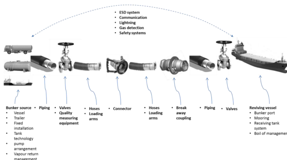
Figura 11. Componenti necessari per il bunkering di GNL in ambito navale
