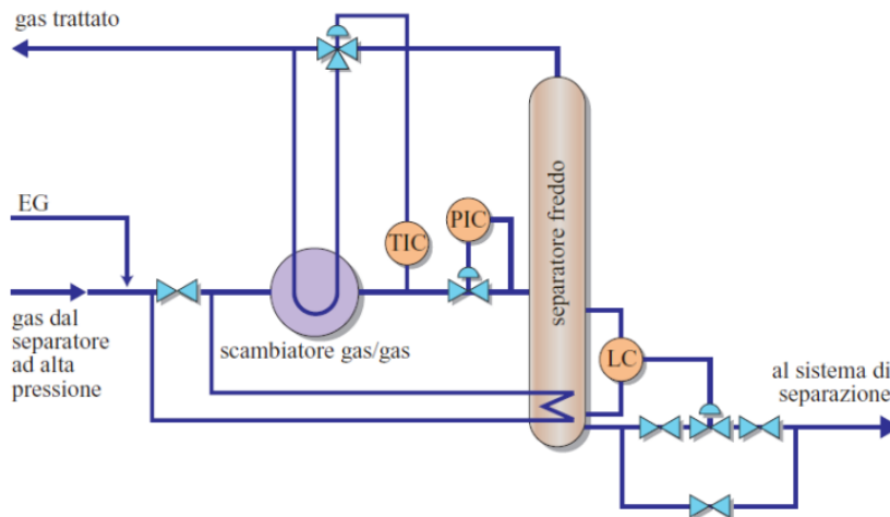
Figura 20. Schema semplificato di impianto a freddo
