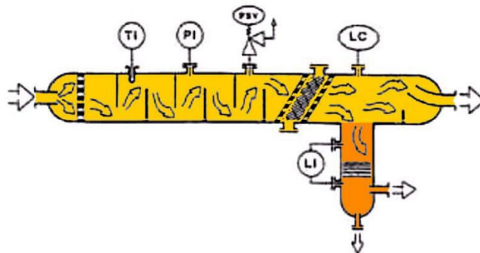
Figura 12. Separatore orizzontale a corpo singolo
