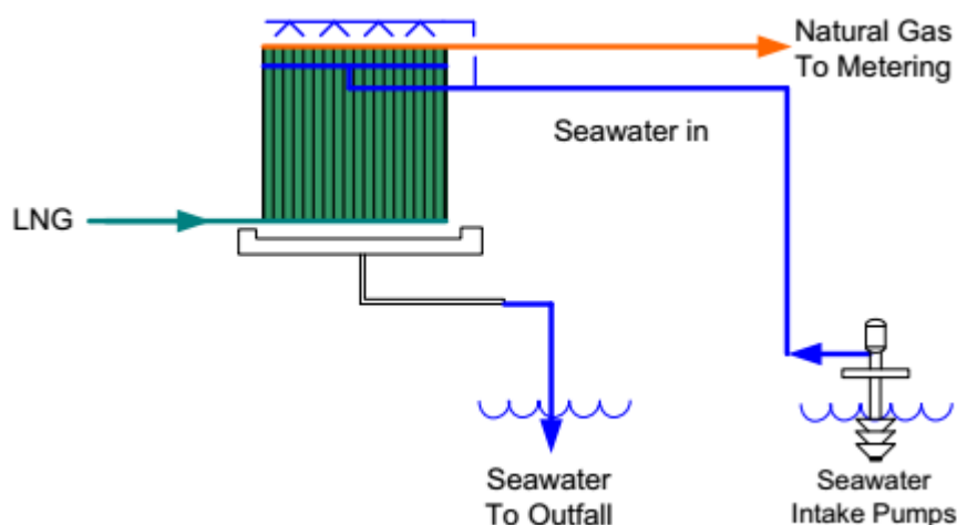
Figura 5 Vaporizzatore Open
