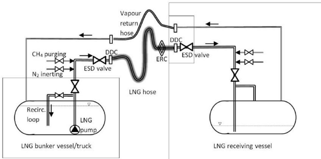
Figura 10. Schema semplificato di linea per il bunkering di GNL
