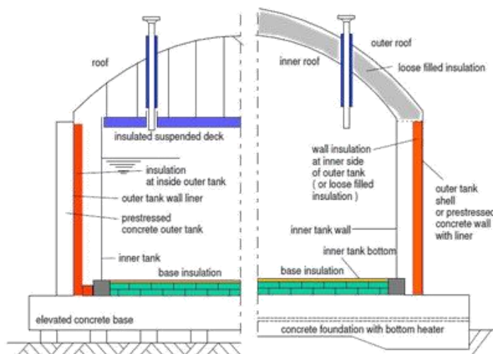
Figura 52. Serbatoio a terra per il bunkering di GNL a contenimento totale
