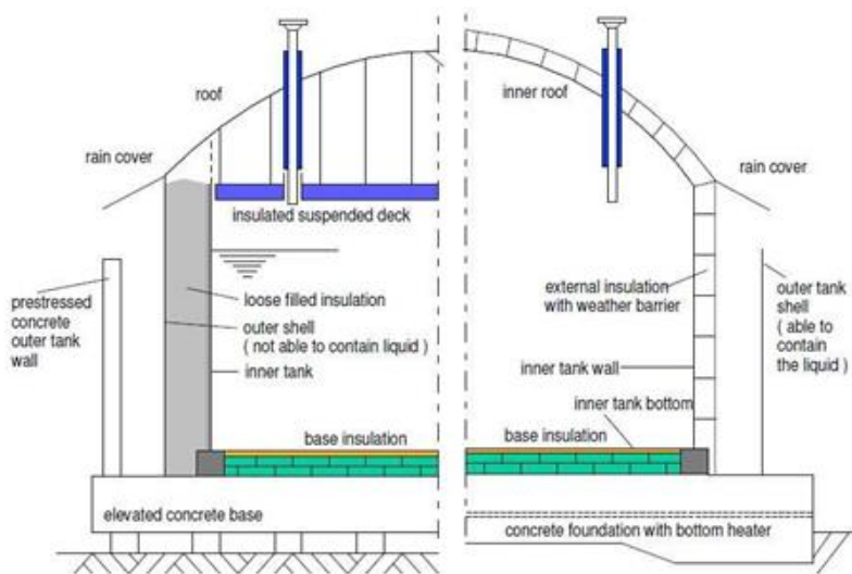
Figura 51. Serbatoio a terra per il bunkering di GNL a doppio contenimento
