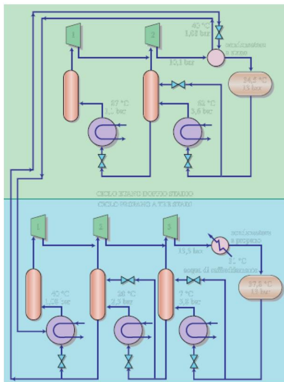
Figura 22. Sistema di refrigerazione in cascata etano (sfondo verde)-propano (sfondo azzurro)
