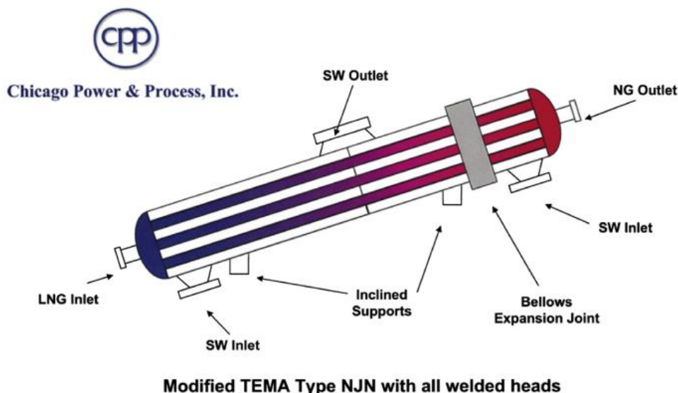
Figura 6 Vaporizzatore a fascio tubiero
