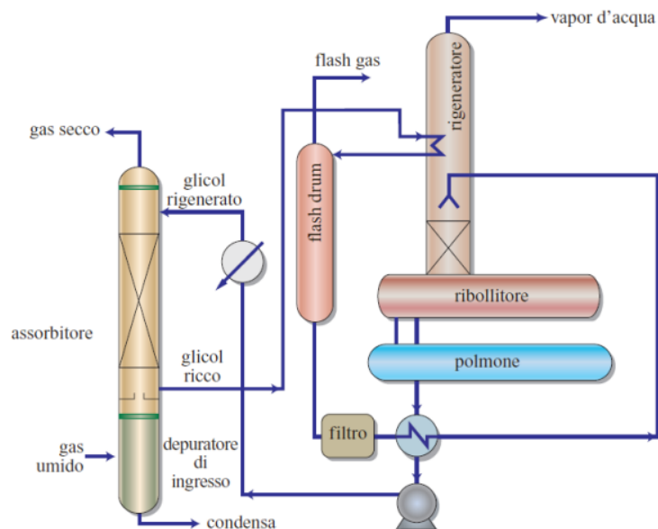
Figura 19. Impianto di disidratazione per assorbimento
