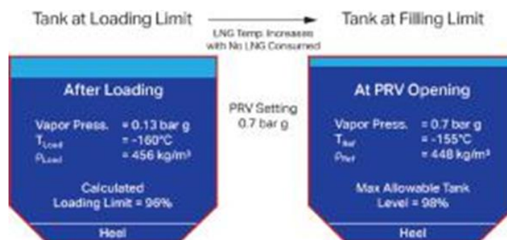
Figura 53. Limite di caricamento per un tipico serbatoio a pressione atmosferica
