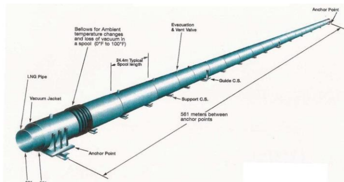
Figura 29. Sistema di piping per il GNL: design con isolamento a vuoto dei tubi
