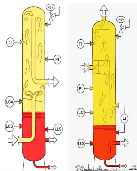
Figura 14: Separatore verticale
