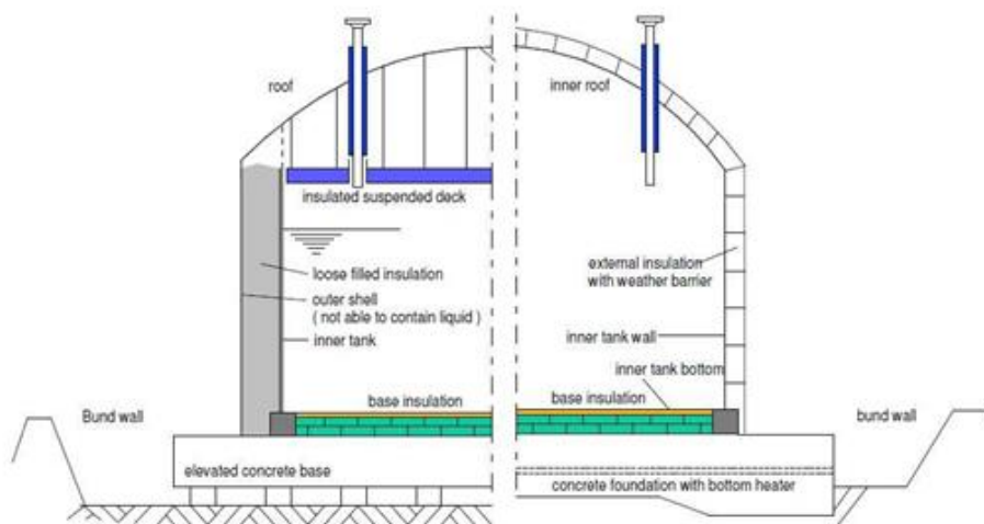
Figura 50. Serbatoio a terra per il bunkering di GNL a singolo contenimento
