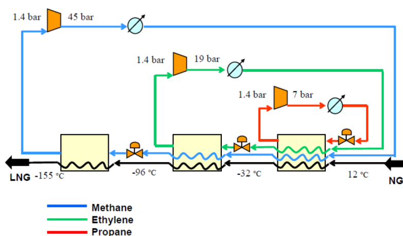
Figura 23. Schema semplificato di un impianto di refrigerazione in cascata a tre stadi
