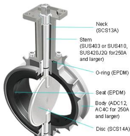
Figura 45. Esempio di valvola a farfalla
