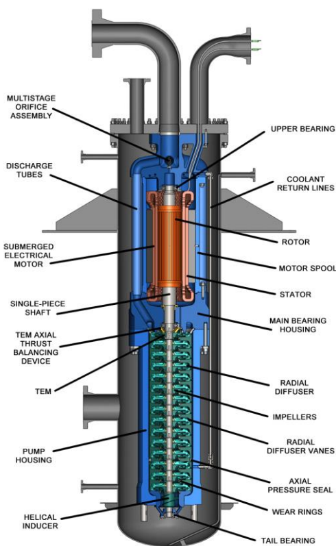
Figura 25. Pompa criogenica per il bunkering di GNL: sezione verticale e indicazione dei componenti
