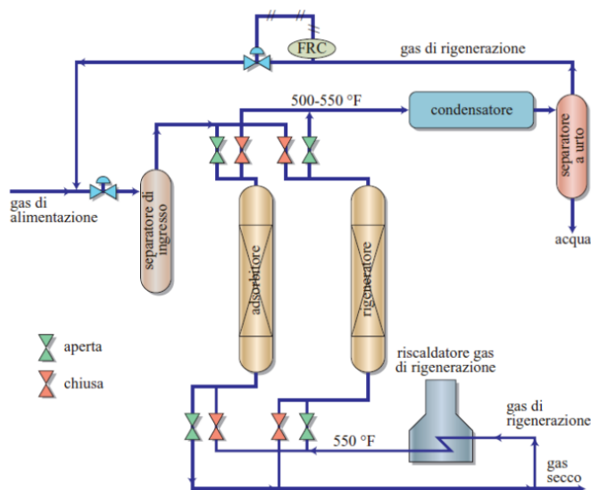
Figura 21. Schema semplificato di un impianto di disidratazione a due letti
