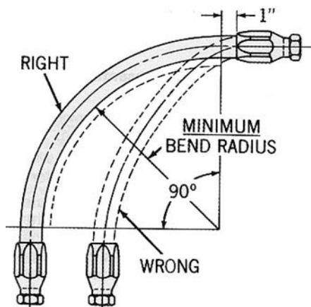
Figura 36. Raggio minimo di curvatura dei tubi flessibili impiegati nel bunkering di GNL
