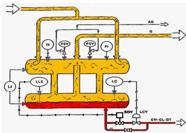
Figura 13. Separatore orizzontale a due corpi
