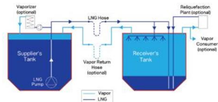
Figura 47. Sistema di gestione del vapore: schema logico
