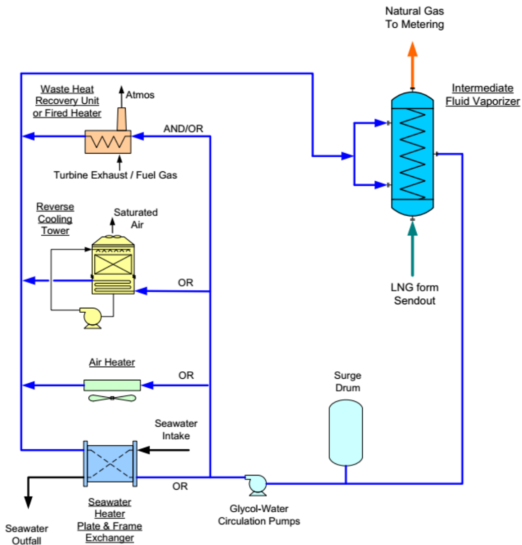
Figura 7 Schema di vaporizzatore a fluido interposto
