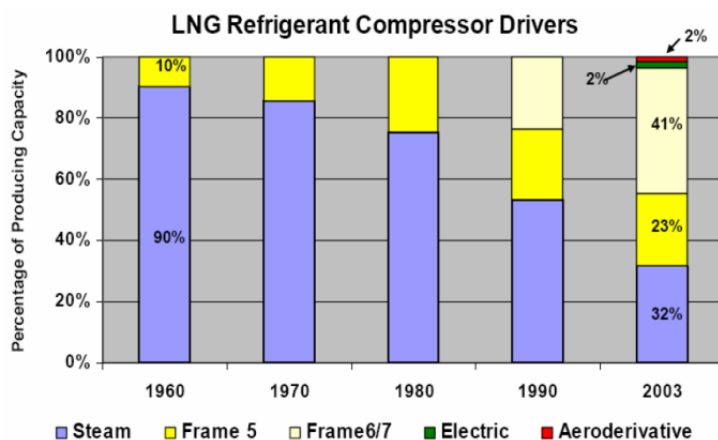
Figura 24: Sistemi di compressione
