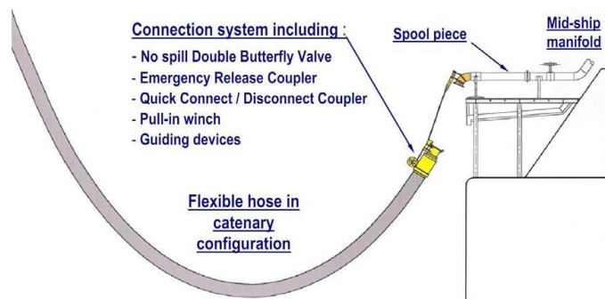
Figura 37. Sistema per la gestione in sicurezza dei tubi flessibili per il bunkering di GNL
