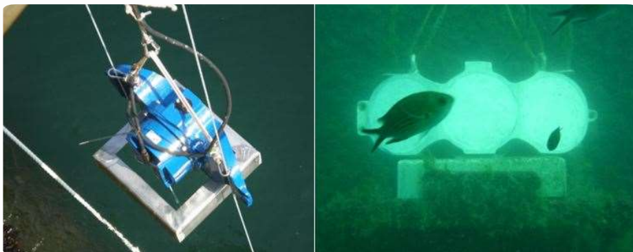
Outils de mesures actuellement installés dans le port de Gênes
