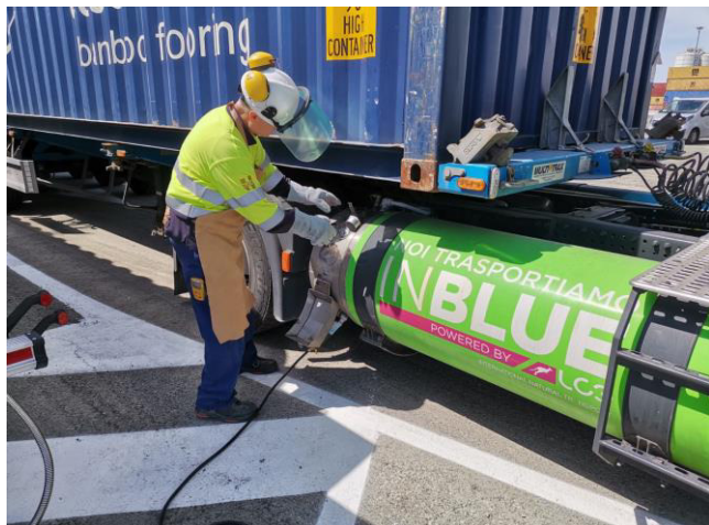
Messa a terra del mezzo e innesto erogatore.
